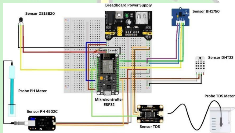
Gambar IV.1 Rangkaian Perangkat Keras ( Hardware )
