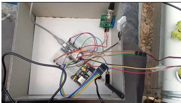
Gambar IV.12 Alat yang sudah dirangkai
