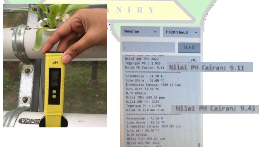
Gambar IV.10 Uji Kalibrasi dengan Air Hidroponik
