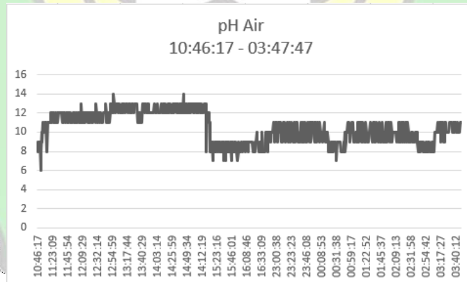
Grafik IV.6 Data Nilai pH Air
