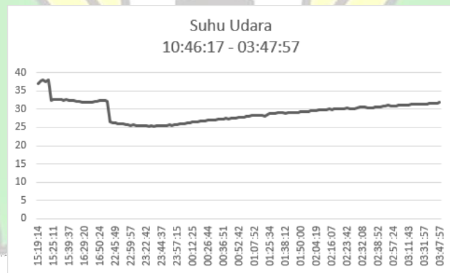
Grafik IV.2 Data Suhu Udara
