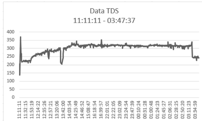
Grafik IV.5 Data Nilai TDS
